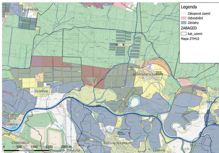
Obr. 5 Přehled závlahově-odvodňovacího systému oblasti Kladruby n. L. zahrnující jak systémy příkopové, tak drenážní. Zdrojem informací je databáze ZVHS (Zemědělská vodohospodářská správa), následně zobrazované v ISMS (Informační systém melioračních staveb), dostupné na adrese https://meliorace.vumop.cz/
