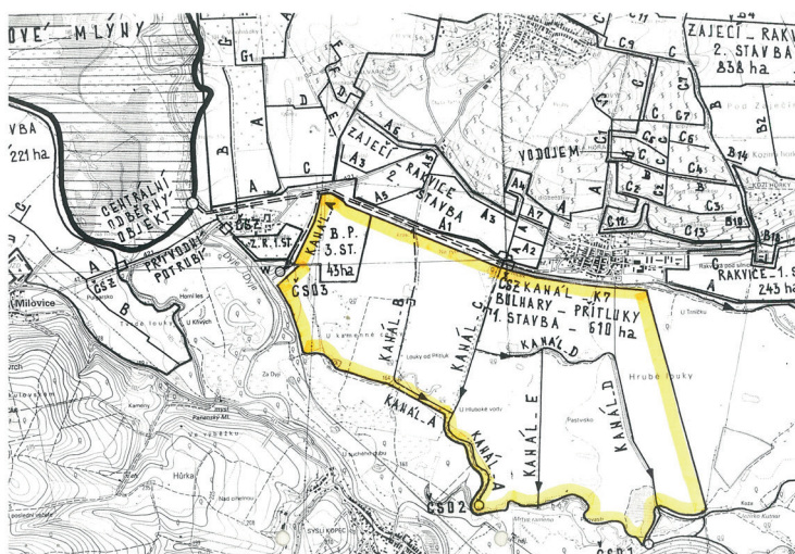
Obr. 3 Výkres projektové dokumentace stavby regulační drenáže Bulhary-Přítluky
