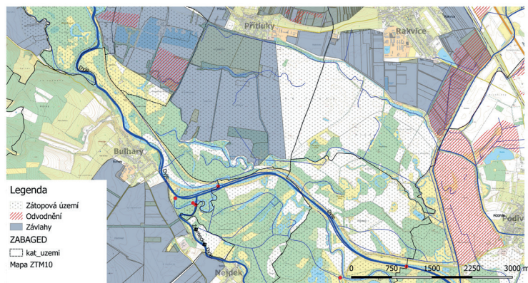
Obr. 2 Závlahová soustava oblasti Bulhary – Přítluky, včetně vybudované stavby regulační drenáže, využívající kombinaci rozvodných příkopů s napojenými závlahově-odvodňovacími dreny
