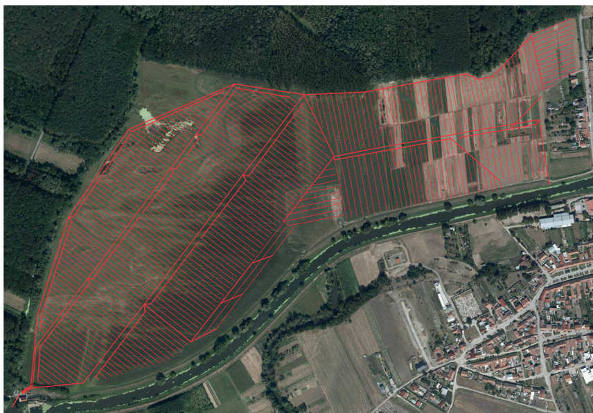
Obr. 4 Situační řešení rozvodné trubní sítě a drénů na lokalitě Uherčice (okr. Břeclav), zobrazena je lokalita 1 s rozlohou 46,5 ha. Zdroj: digitalizovaná situace projektové dokumentace na pozadí leteckého snímku (Mapy.cz)
